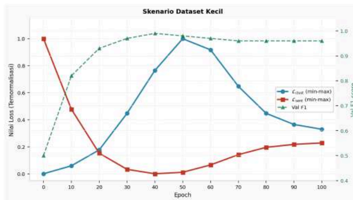
Gambar 4.3: Skenario dataset kecil: L_{sent} mencapai kondisi stabil lebih dahulu, kemudian L_{clust} mulai menurun dan kedua komponen menunjukkan pola yang lebih seimbang.
