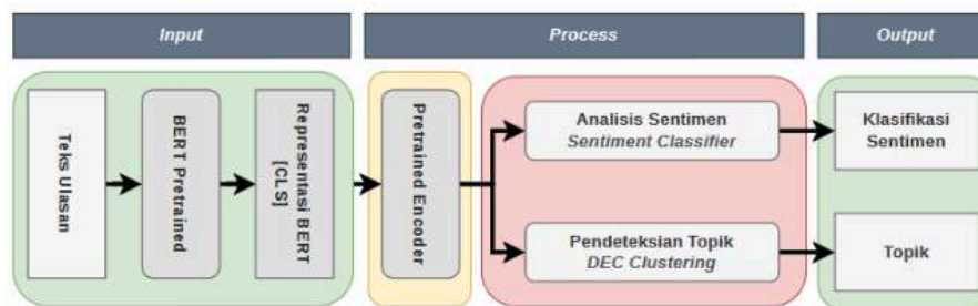
Gambar 3.1: Alur metode analisis sentimen dan pendeteksian topik
