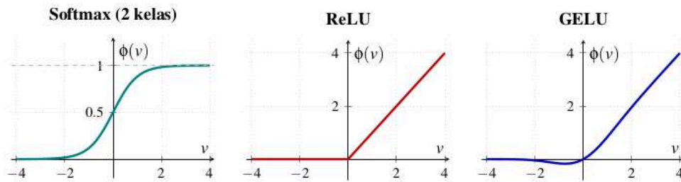
Gambar 2.4: Grafik fungsi aktivasi: Softmax , ReLU, dan GELU
